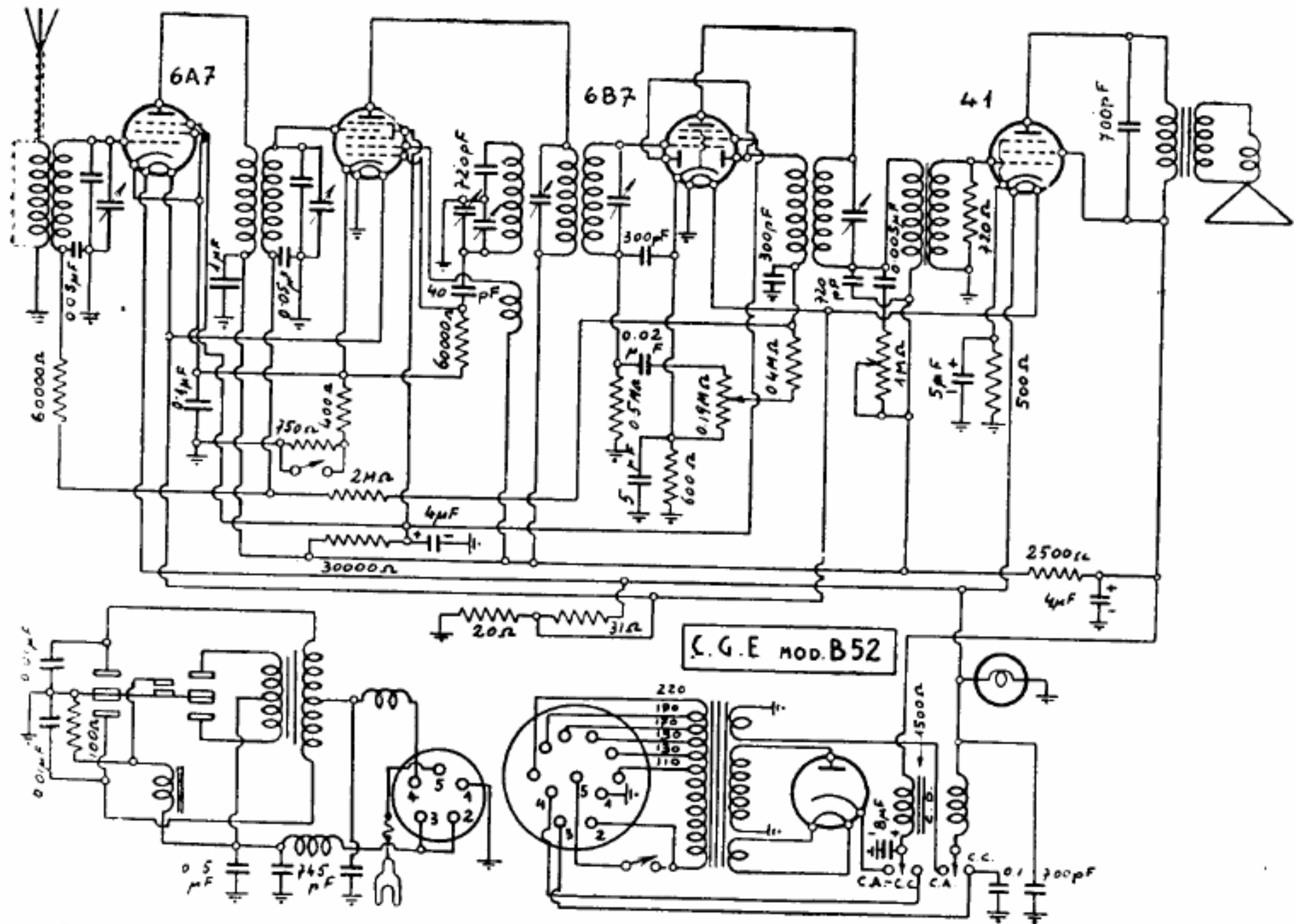
COMPAGNIA GENERALE DI ELETTRICITÀ. — Mod. « B 52 Auto ». - Produzione 1936. - Media frequenza: 175 kHz.
